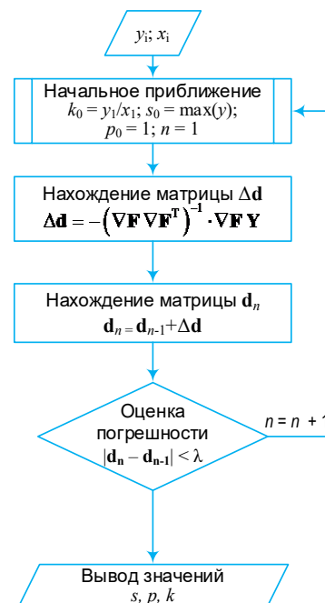
Рис. 6. Блок-схема алгоритма выбора параметров модели
