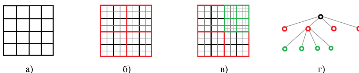
Рисунок. Дерево квадратов с использованием сетки 4 \times 4
