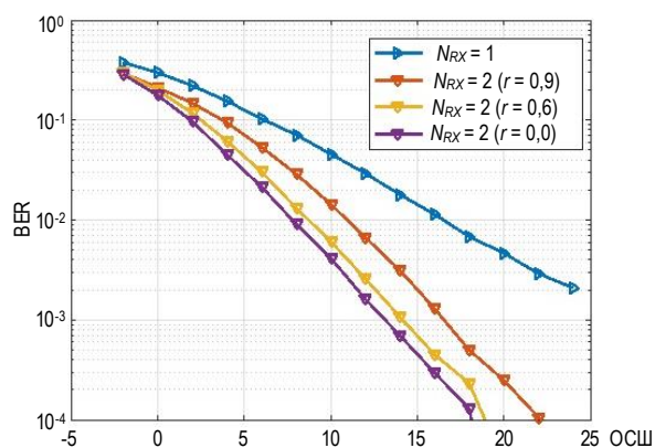
Рис. 5. Зависимость BER от отношения сигнал / шум
