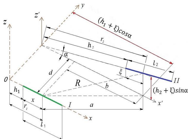
Рис. 1. Оси произвольно расположенных проводников в двух параллельных плоскостях
