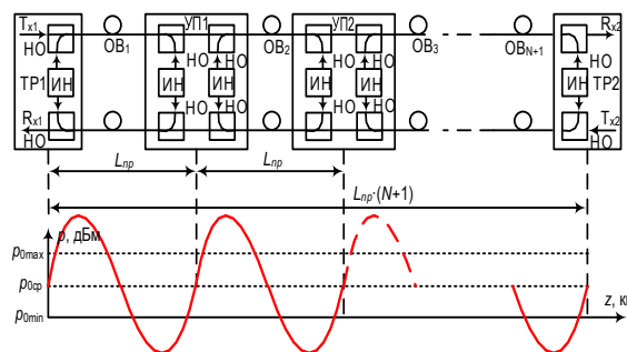
Рис. 8. Схема линейного тракта ВОСС с РА и двунаправленной накачкой
