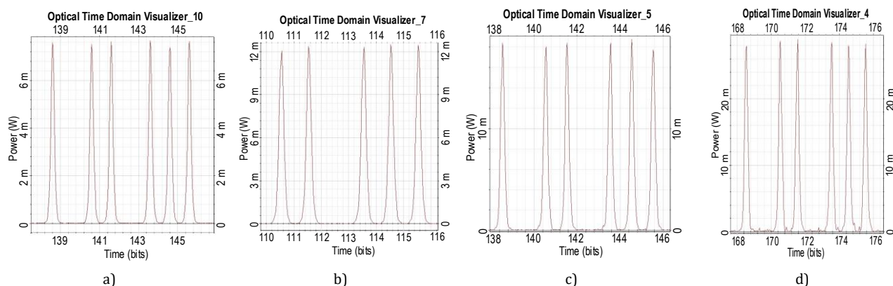
Рис. 7. Форма импульсов на выходах многопролетных квазисолитонных ВОСС: длина 50 км × 10 = 500 км (а); 75 км × 7 = 525 км (b); 100 км × 5 = 500 км (с); 125 км × 4 = 500 км (d)
