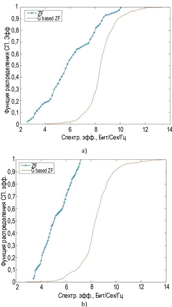
Рис. 1. Распределение СЭ при прекодировании ZF и выборе абонентов SUS, число обусловленности канала CN = 240 (a) и CN = 500 (b)
