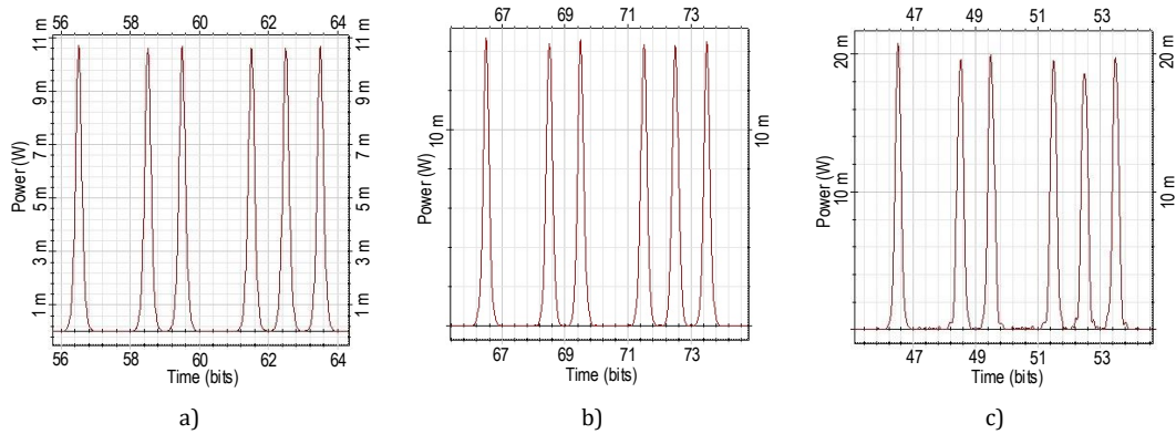
Рис. 3. Форма импульсов на выходах многопролетных квазисолитонных ВОСС: длина 50 км × 10 = 500 км (а); 75 км × 6 = 450 км (б); 100 км × 4 = 400 км (с)
