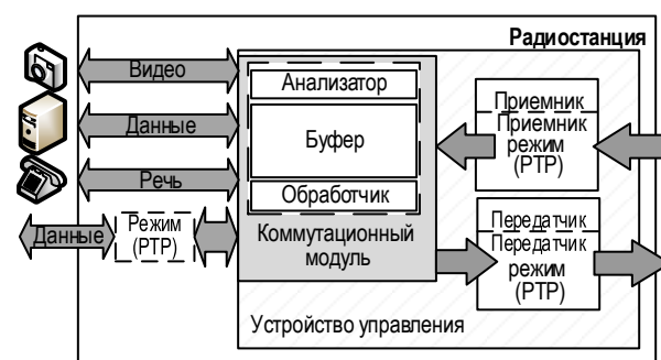
Рис. 2. Вариант функциональной схемы элемента радиосвязи
