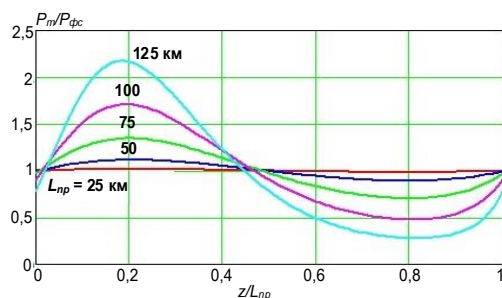
Рис. 9. Зависимости нормированной относительной мощности p(z) от относительного расстояния z/L_{np} в пределах одного УУ
