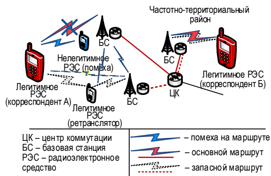
Рис. 1. Вариант построения самоорганизующейся сети радиосвязи
