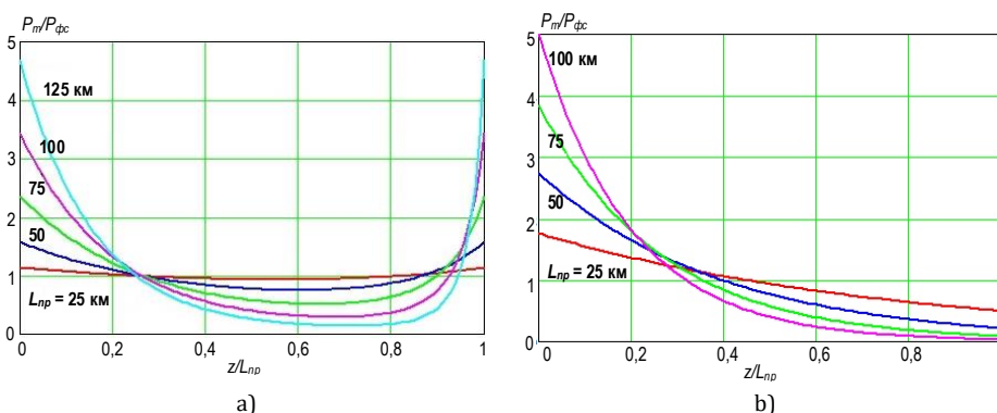
Рис. 5. Зависимости нормированной относительной мощности p_n(z) от относительного расстояния z/L_{np} в пределах одного УУ: для РА с встречной накачкой (а); дискретных EDFA (б)
