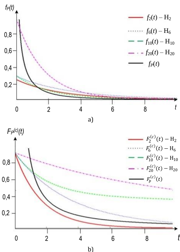
Рис. 3. Графики аппроксимации распределения Парето: а) плотность; б) дополнительная интегральная функция
