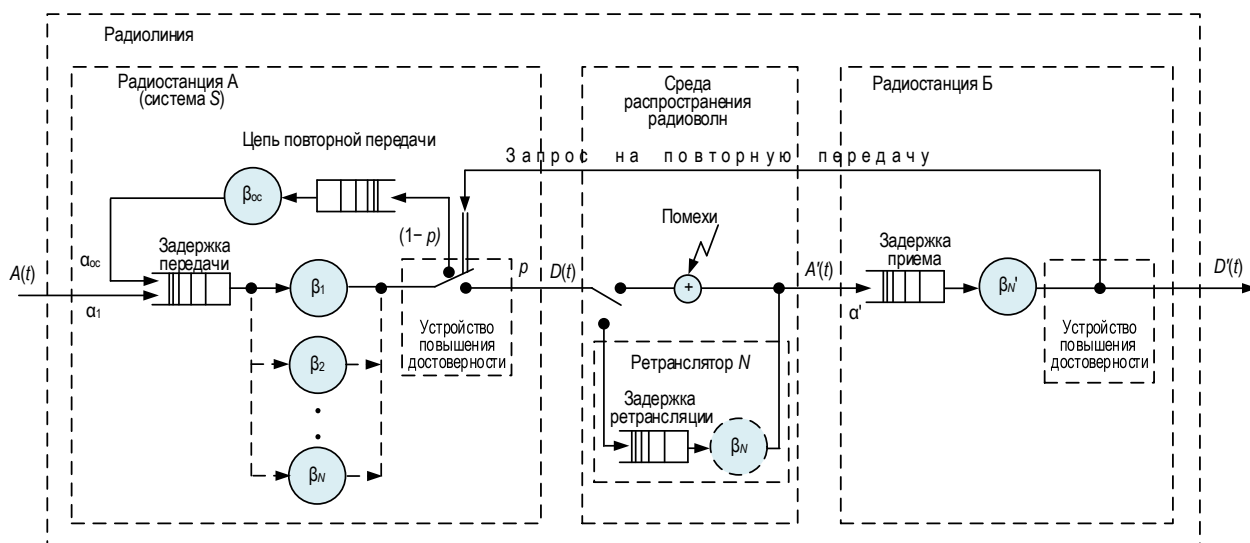
Рис. 3. Модель радиосвязи в ССПО
