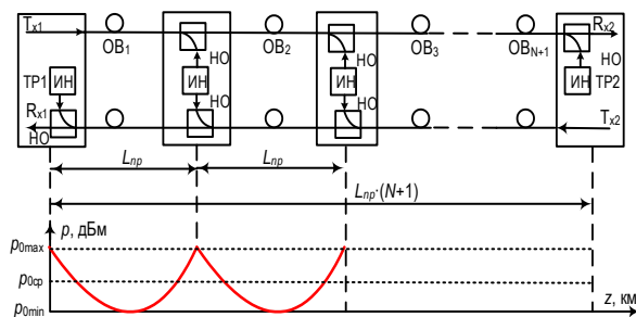
Рис. 4. Схема линейного тракта ВОСС с РА и встречной накачкой
