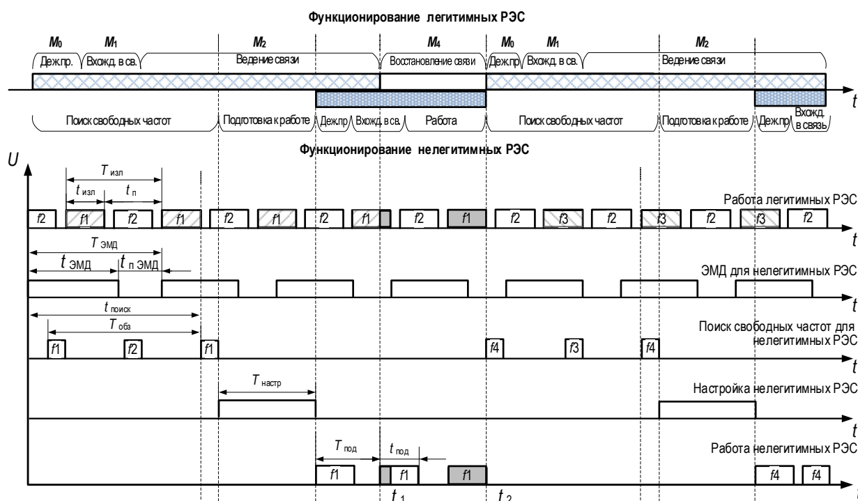
Рис. 6. Временная диаграмма функционирования РЭС
