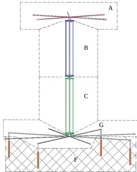
Рис. 2. Схематическое изображение НВВТП в общем виде Fig. 2. Schematic Representation of the Unbalanced Monopole with Shunt Feed
