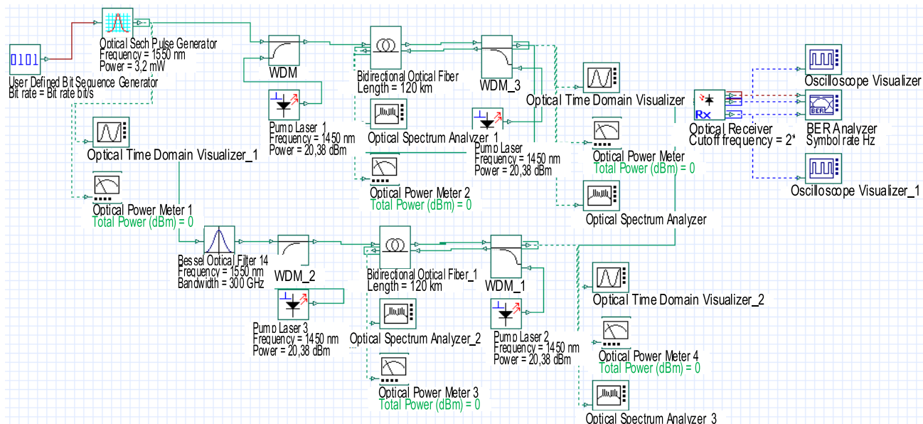
Рис. 10. Схема из двух последовательно соединенных пролетов
