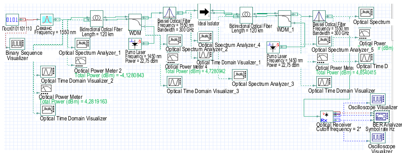
Рис. 6. Схема из двух последовательно соединенных УУ
