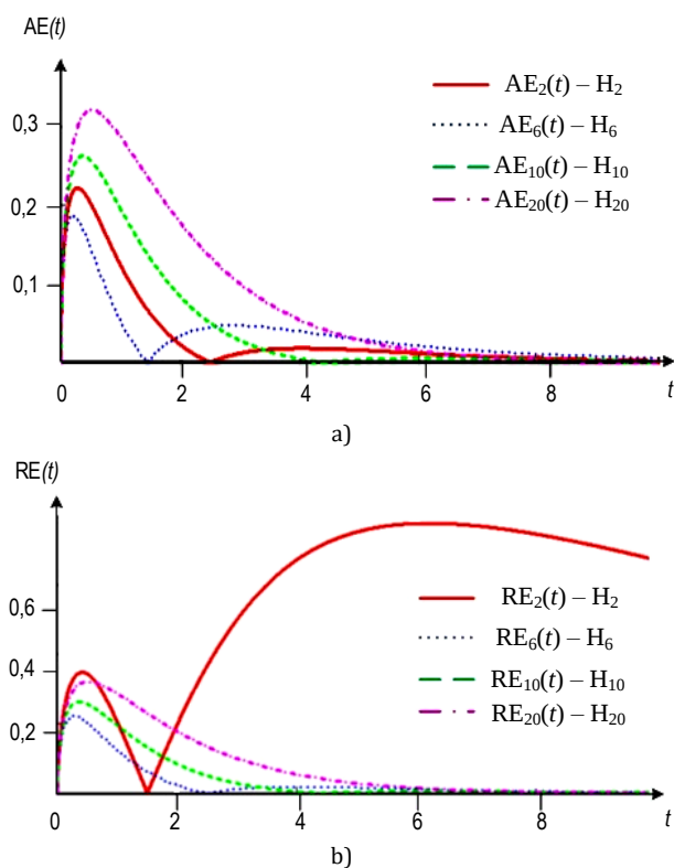
Рис. 2. Ошибка аппроксимации распределения Вейбулла: а) абсолютная; б) относительная
