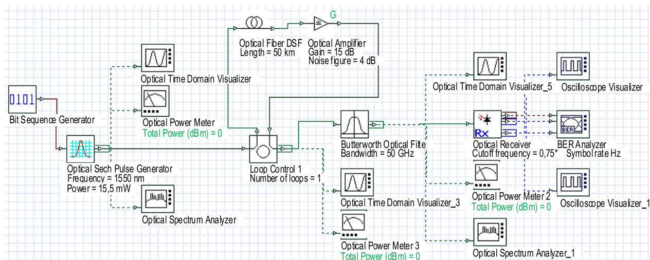
Рис. 2. Схема моделирования многопролетной квазисолитонной ВОСС с дискретными ОУ
