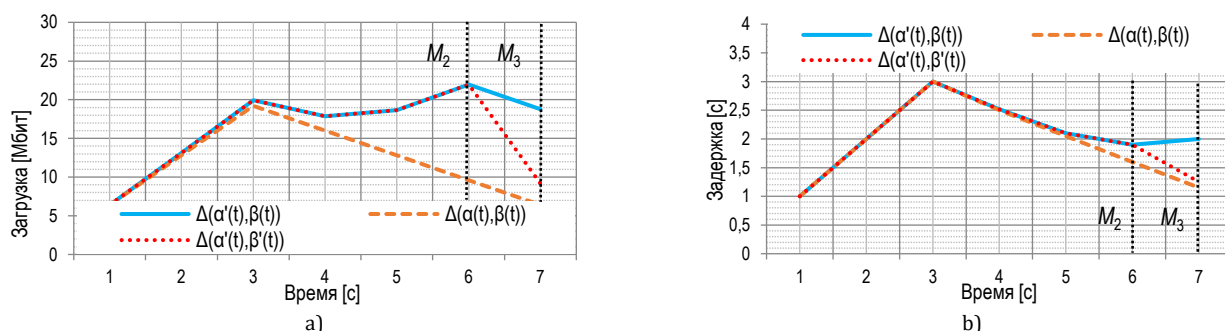
Рис. 9. Зависимость а) задержки и б) загрузки от времени моделирования радиолнии в ССПО
