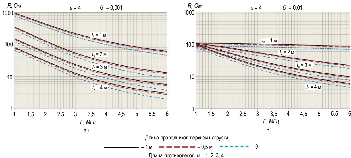
Рис. 4. Вещественная составляющая сопротивления потерь НВВТП в зависимости от частоты для влажной (а) и сухой (б) почв
