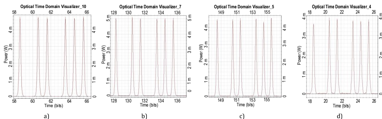
Рис. 11. Форма импульсов на выходах многопролетных квазисолитонных ВОСС: длина 50 км × 10 = 500 км (a); 75 км × 7 = 525 км (b); 100 км × 5 = 500 км (c); 125 км × 4 = 500 км (d)
