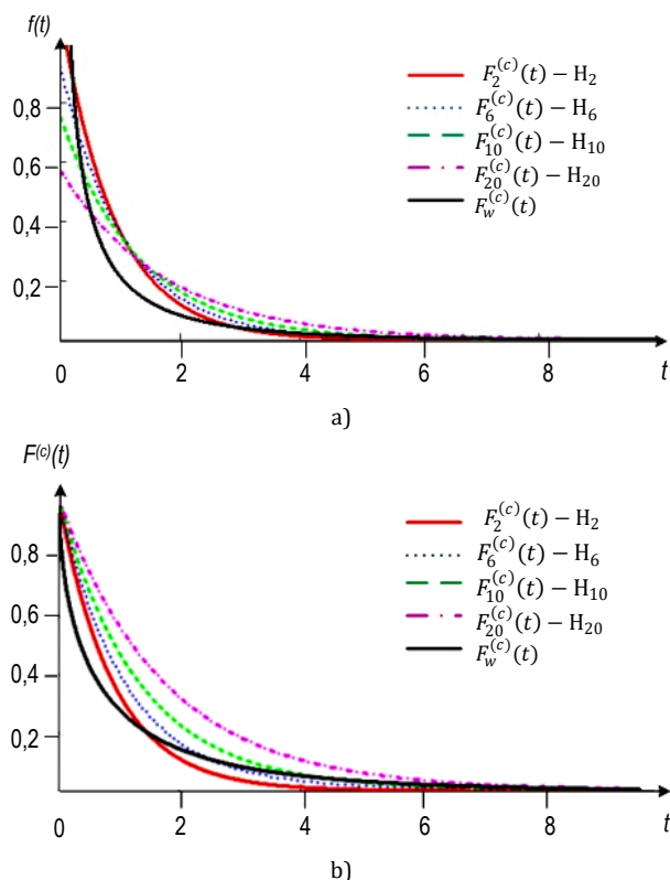
Рис. 1. Графики аппроксимации распределения Вейбулла: а) плотность; б) дополнительная интегральная функция
