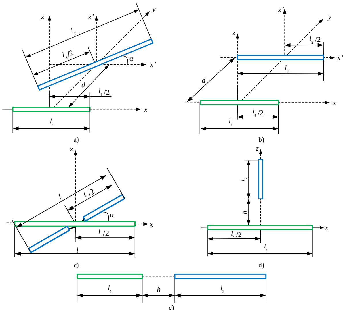
Рис. 3. Возможные пары проводников в конструкции НВВТП
