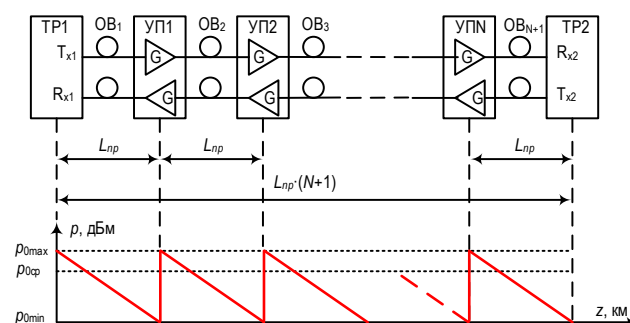
Рис. 1. Схема линейного тракта ВОСС с дискретными ОУ
