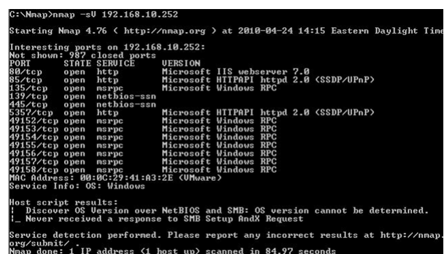
Рис. 1. Реакция Honeyrot, имитирующая открытые порты MS Windows при сканировании с помощью nmap
