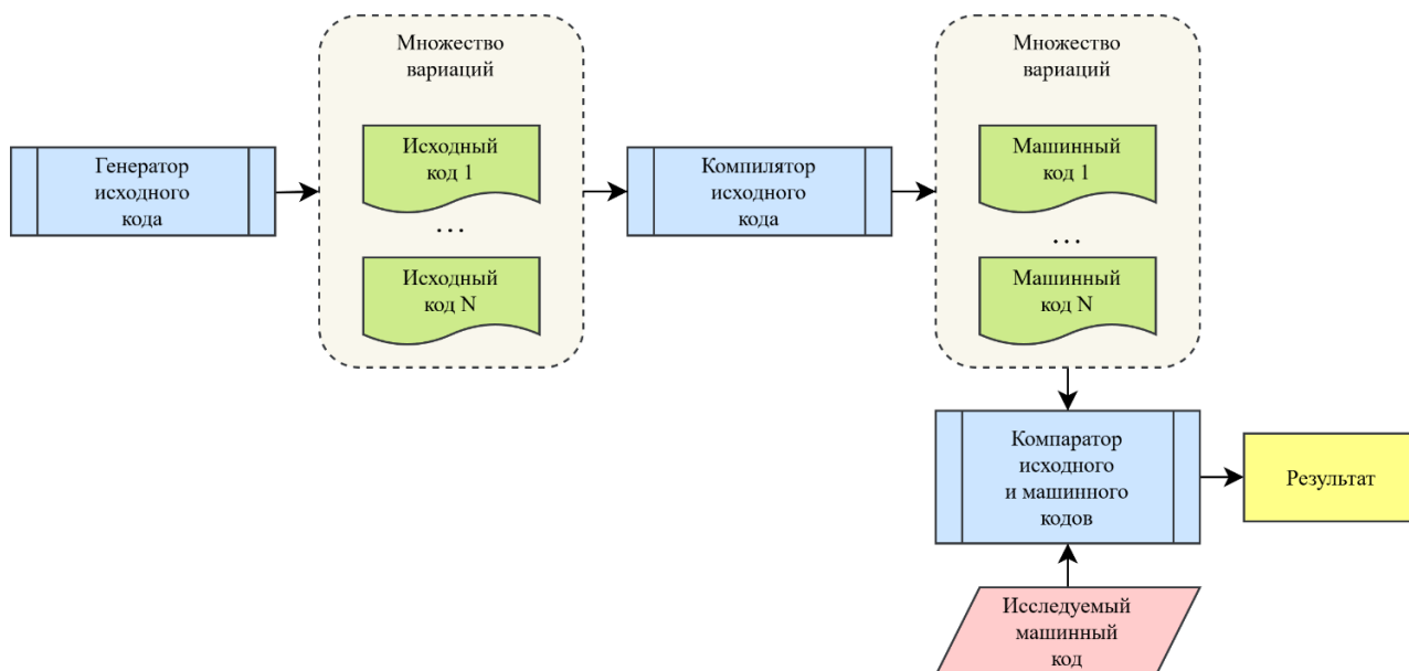
Рис. 1. Схема проведения реверс-инжиниринга путем генерации вариаций исходного кода
