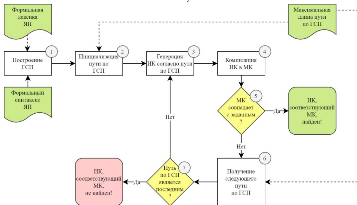
Рис. 3. Схема работы Метода с функционалом для реверс-инжиниринга
