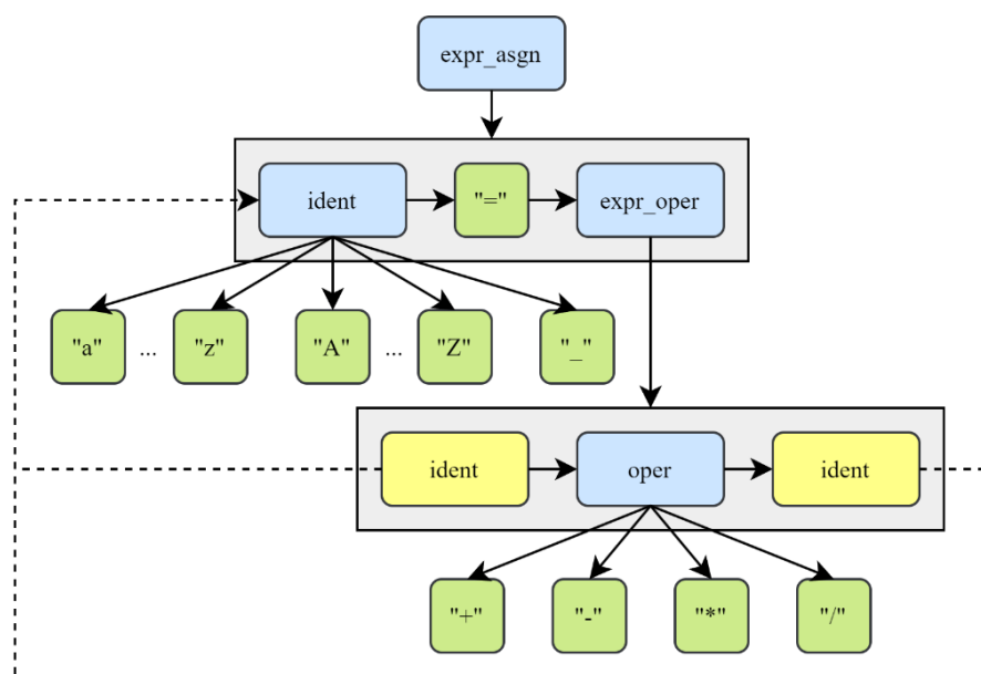
Рис. 4. Представление графа синтаксических правил для Листинга
