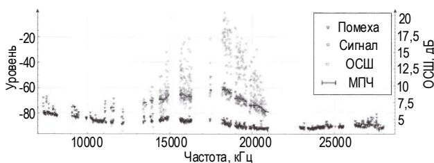
Рис. 1. Ионограмма трассового зондирования на частотах, выделенных для радиоперехвата
