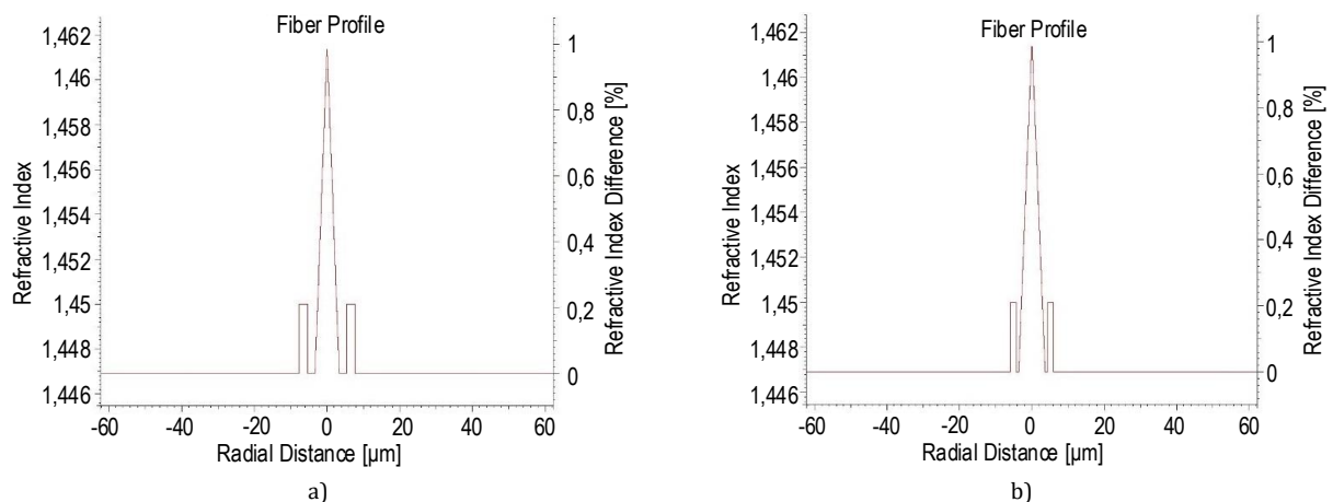
Рис. 5. ППП ОМ ОВ с ДГС 4,5 пс²/км (а) и -4,5 пс²/км (б)
