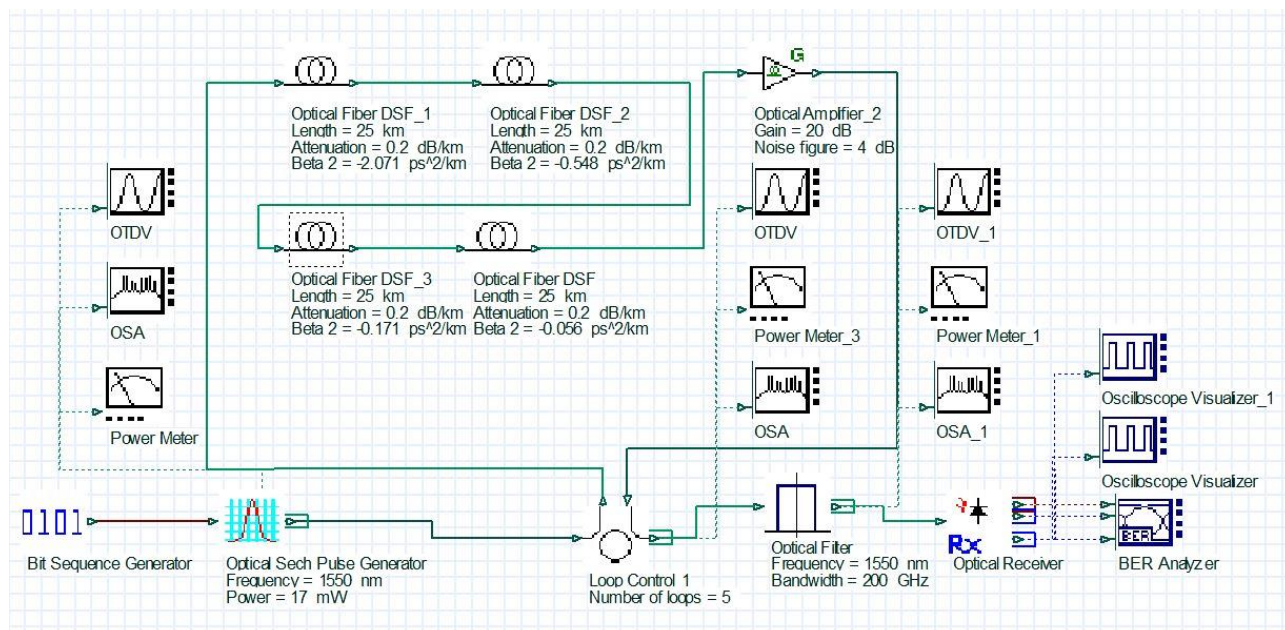
Рис. 3. Схема квазисолитонной многопролетной ВОСС с управлением дисперсией
