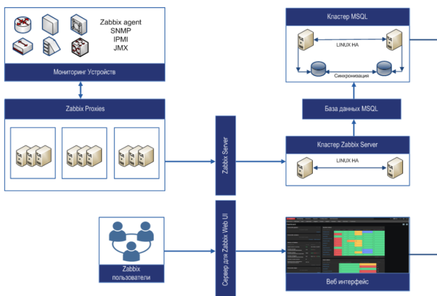
Рис. 1. Обобщенная структурная схема универсальной сети мониторинга
