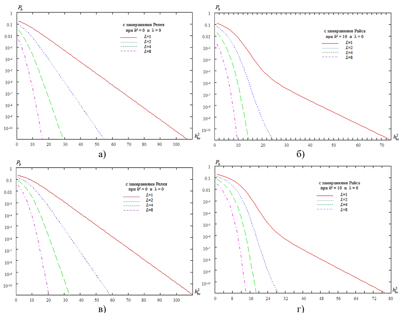
Рисунок 1. Зависимость вероятности средней битовой ошибки от отношения сигнал/шум при пространственном разнесенном приеме:
