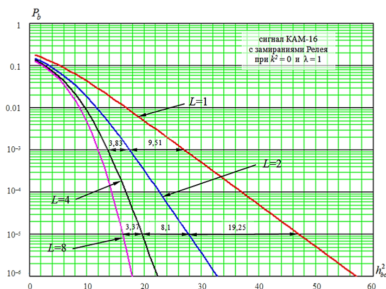
Рисунок 2. Зависимость вероятности средней битовой ошибки от отношения сигнал/шум при частотном разнесенном приеме сигнала КАМ164 и релейскими замираниях
