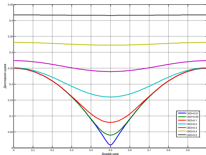
Рисунок 2. Дисперсия случайного процесса на выходе АЦП в зависимости от дрейфа нуля при различных СКО теплового шума
