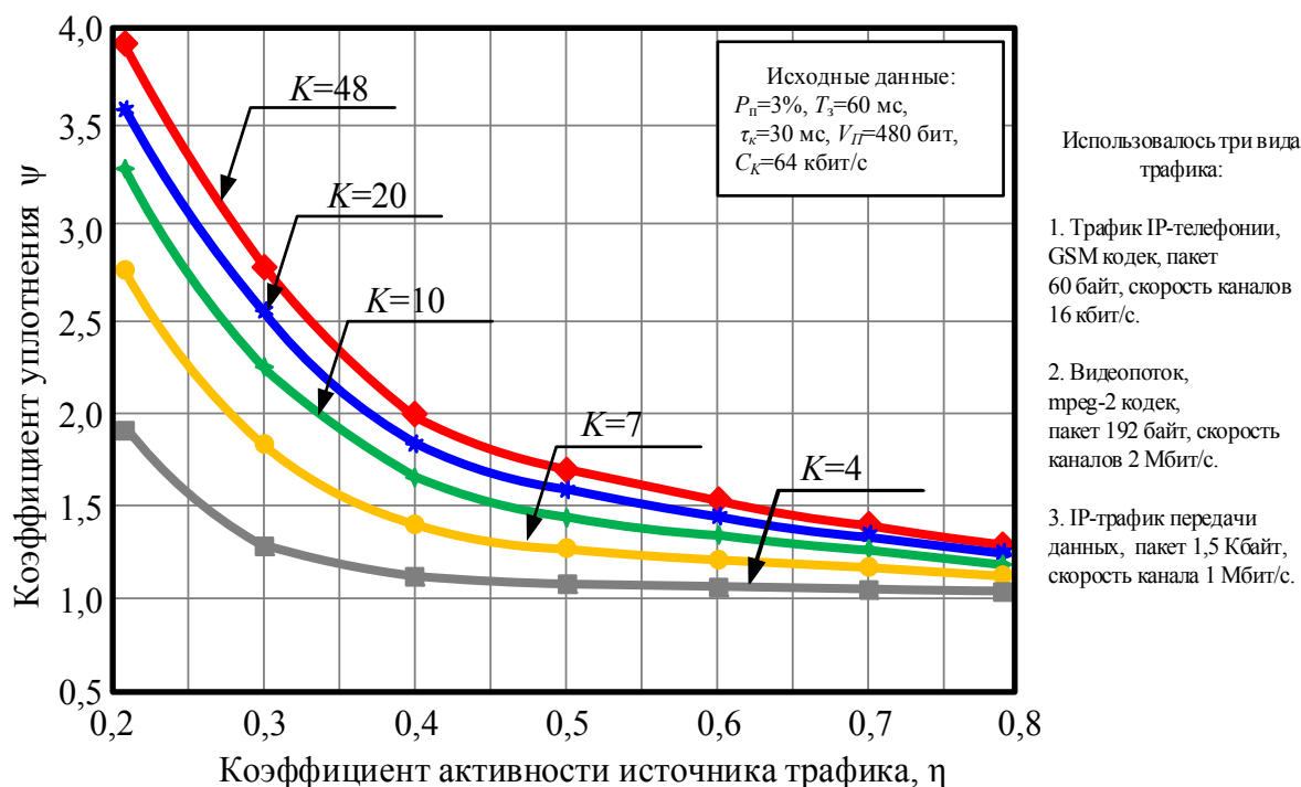
Рисунок 6. Зависимость коэффициента уплотнения от активности источников трафика при изменении канальной емкости мультимплексора
