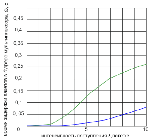
Зависимость времени задержки пакетов от интенсивности поступления пакетов
