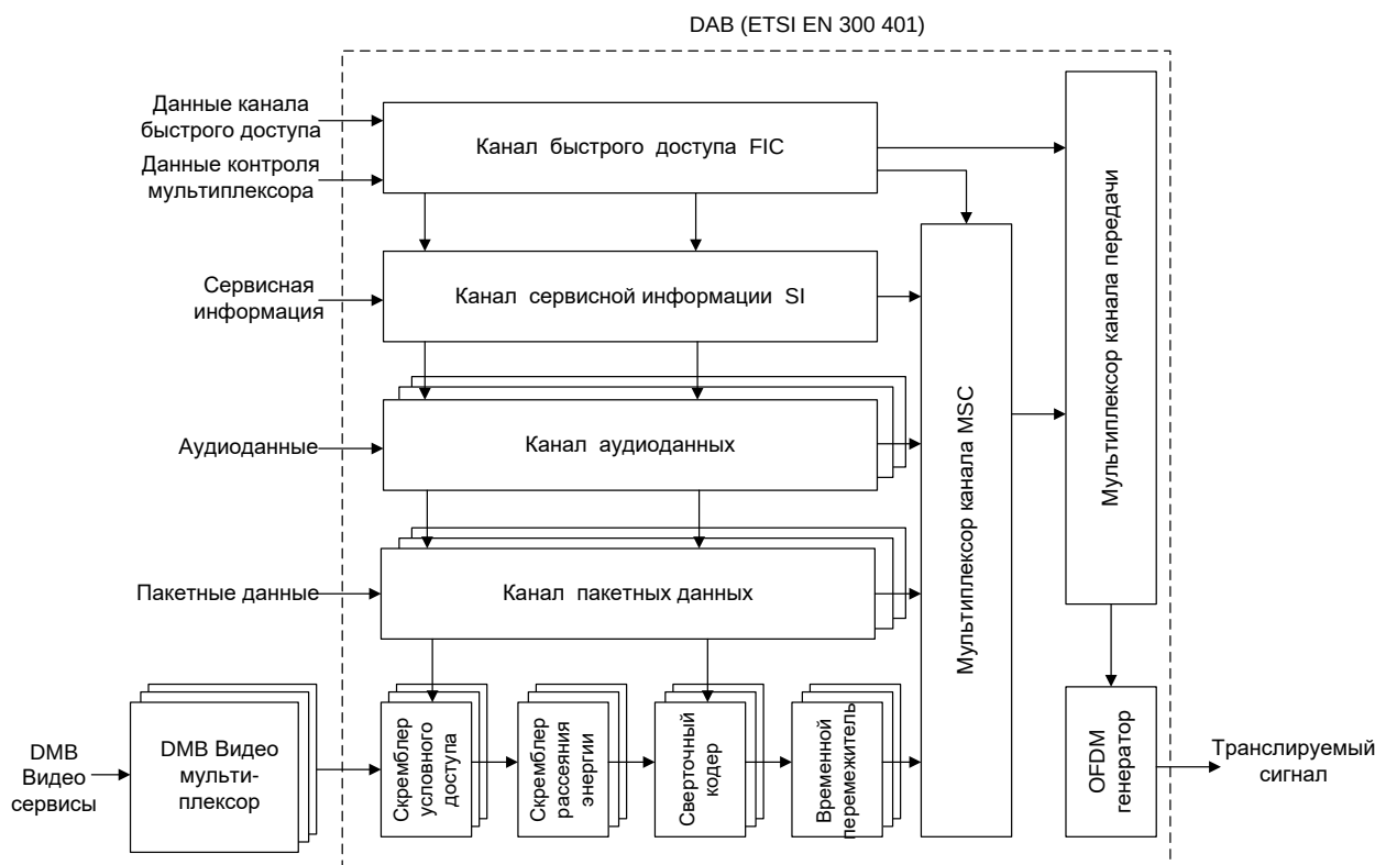
Рис. 5. Увеличенная структурная схема системы DAB с возможностью передачи видеoinформации (T-DMB)
