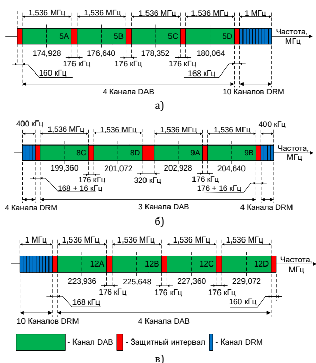
Рис. 4. Совместная передача мультимплексов DAB и DRM+ в полосе частот 174...230 МГц в радиоканале шириной 8 МГц: а) 6-й ТВК; б)
