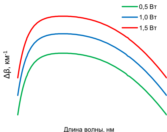
Рис. 7. Спектральная зависимость фазовой расстройки для первой высшей моды микроструктурированного световода с сердцевинной диаметром 8 мкм
