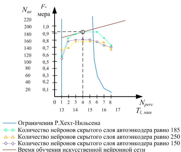
Рис. 4. Зависимости значений показателя F -мера и продолжительности обучения от структуры комбинированной искусственной нейронной сети
